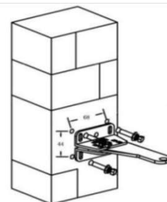
Монтаж при бетонови колони
