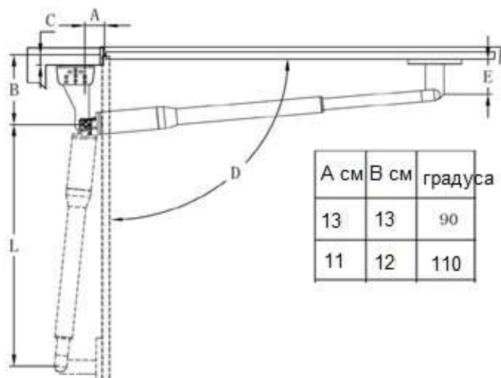
Схеми на размерите А и В
