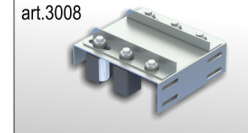
Piastra regolabile 4 olive/ Adjustable upper plate 4 rollers art.3008
